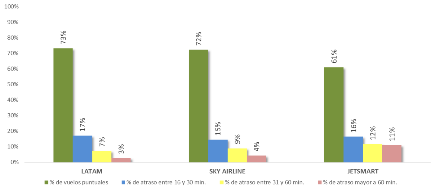
Gráfico 5: Detalle puntualidad de líneas aéreas en despegues nacionales desde Temuco
