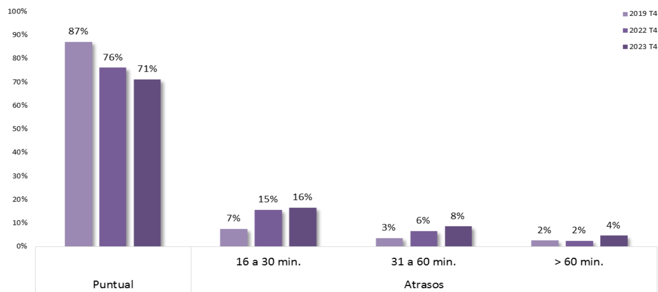
Gráfico 3: Evolución puntualidad en despegues IV trimestre desde Temuco en rutas nacionales
